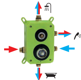
SCHÉMA ZAPOJENÍ TŘÍCESTNÉHO BOXU
